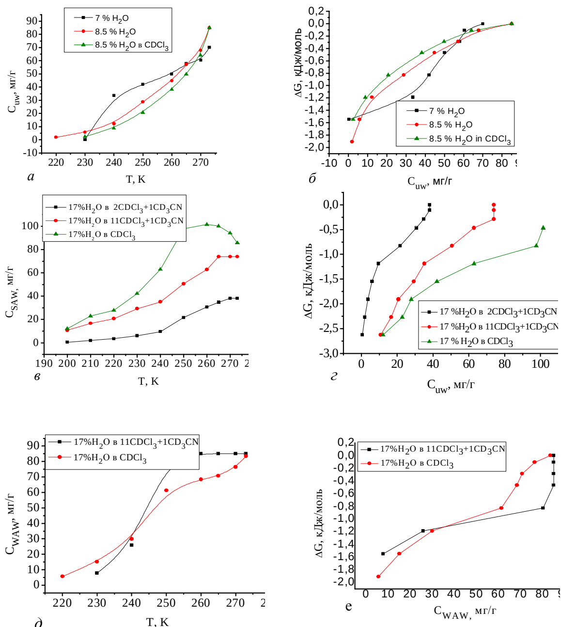
Рис. 10. Температурные зависимости концентрации незамерзающей воды (а, в, д) и зависимости изменения свободной энергии Гиббса (б, г, е) для композита ГЖА с гидратированностью 7 и 8,5 % мас. (а, б), и 17 % мас. (в-е).
