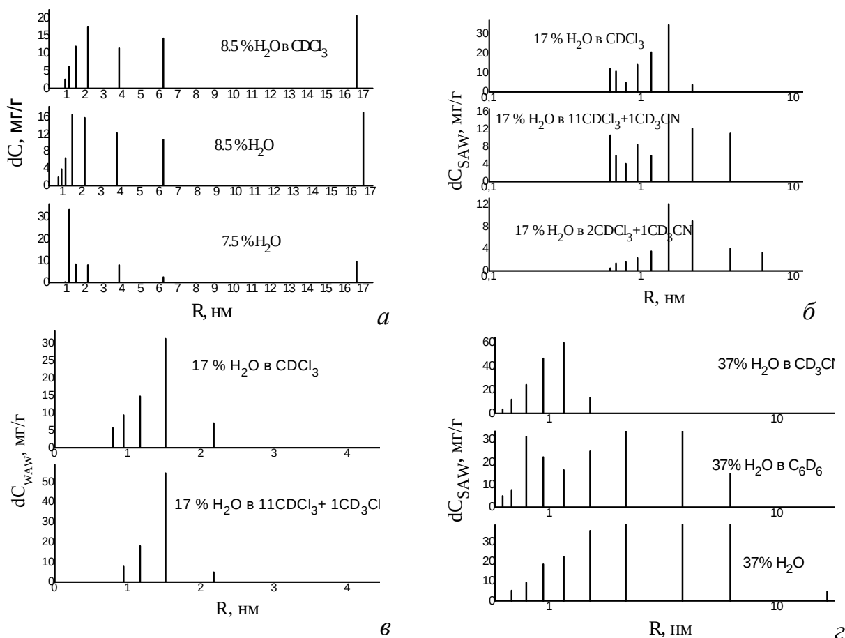
Рис. 12. Распределение по размерам водных структур в гидратированных нанокомпозитах ГЖА в воздушной и органической средах для C_{H_2O} 7 и 8,5 % мас. (а); 17 % мас. (б, в), 37 % мас. (з).
